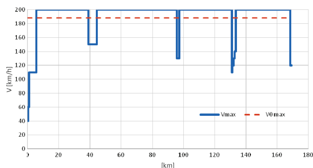
Rys. 2. Profil prędkości maksymalnej na linii Hanower – Hamburg-Harburg: (jako V_{0 \max} zaznaczono wartość średniej ważonej prędkości maksymalnej obliczonej jako średnia harmoniczna) [opracowanie własne]
