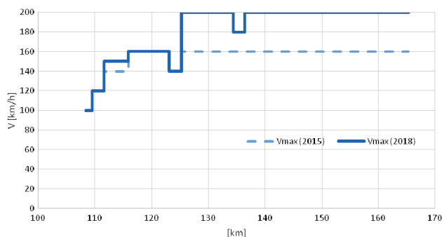
Rys. 4. Profil prędkości maksymalnej linii Halle – Bebra na odcinku Erfurt – Eisenach [opracowanie własne]
