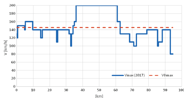
Rys. 3. Profil prędkości maksymalnej na linii (Norymberga-) Fürth – Würzburg [opracowanie własne]
