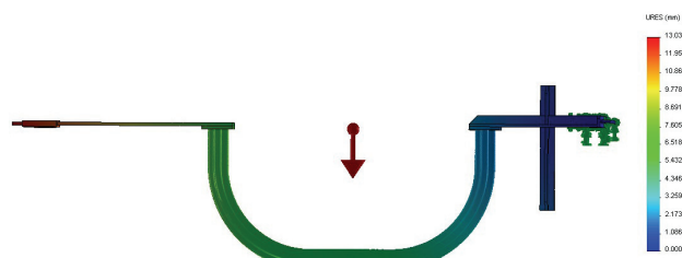
Rys. 10. Wyniki uzyskane z symulacji przemieszczeń poszczególnych punktów elementów przyrządu zamocowanego na końcu przyrządu pomiarowego od strony przeciwnej do zespołu pomiarowego poziomo wybrzuszeniem kabłąka do dołu, wariant A przekroju kabłąka [opracowanie własne]
