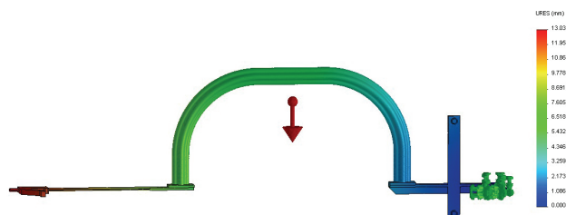
Rys. 9. Wyniki uzyskane z symulacji przemieszczeń poszczególnych punktów elementów przyrządu zamocowanego na końcu przyrządu pomiarowego od strony przeciwnej do zespołu pomiarowego poziomo wybrzuszeniem kabłąka do góry, wariant A przekroju kabłąka [opracowanie własne]
