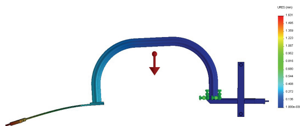
Rys. 5. Wyniki uzyskane z symulacji przemieszczeń poszczególnych punktów elementów przyrządu zamocowanego na końcu kabłąka przyrządu pomiarowego od strony przeciwnej do zespołu pomiarowego poziomo wyrzusem kabłąka do góry, wariant A przekroju kabłąka [opracowanie własne]
