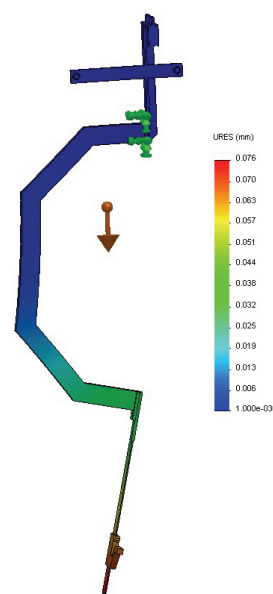
Rys. 11. Wyniki uzyskane z symulacji przemieszczeń poszczególnych punktów elementów przyrządu zamocowanego na końcu kabłąka przyrządu pomiarowego od strony przeciwnej do zespołu pomiarowego pionowo zespołem pomiarowym do dołu, wariant B przekroju kabłąka [opracowanie własne]
