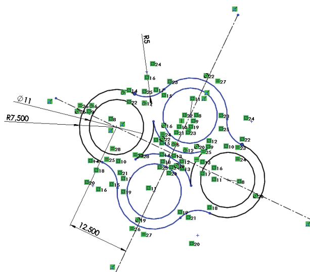
Rys. 1. Przekrój kabłąka przyrządu do pomiaru średnicy okręgu tocznego kół zestawów kołowych zbudowany ze spawanych czterech rurek cienkościennych (wariant A przekroju) [opracowanie własne]
