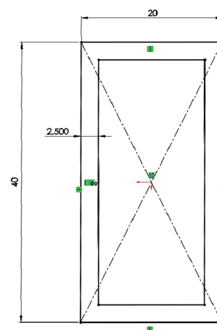
Rys. 2. Prostokątny przekrój kabłąka przyrządu do pomiaru średnicy okręgu tocznego kół zestawów kołowych (wariant B przekroju) [opracowanie własne]
