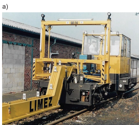
Rys. 7. Pojazd pomiarowy LIMEZ I: a) widok ramy z przyrządami pomiarowymi, b) widok pojazdu [fot. ze zbioru autora]
