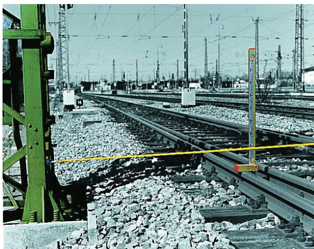
Rys. 3. Przykłady ręcznego pomiaru ograniczeń skrajniowych: a) położenie słupa trakcyjnego [12], b) położenie tarczy semafora [fot. Deutsche Bahn AG, Geschäftsbereich Netz]
